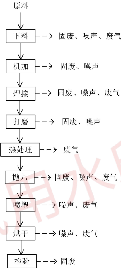
图 2-2 钢结构类试验台工艺流程及产污环节图
