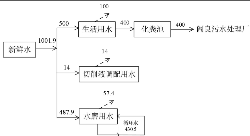
图 2-1 扩建后全厂水平衡图
