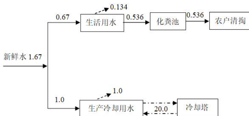
图 2 水平衡图（单位：m 3 /d）
